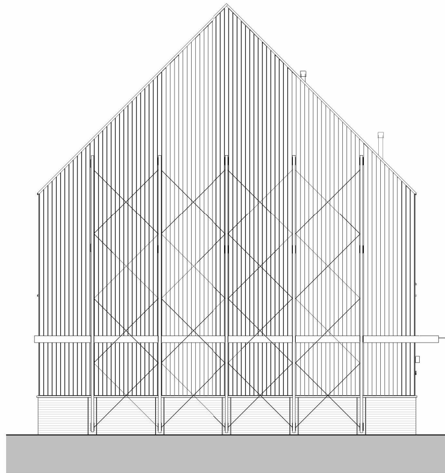
kopgevel
