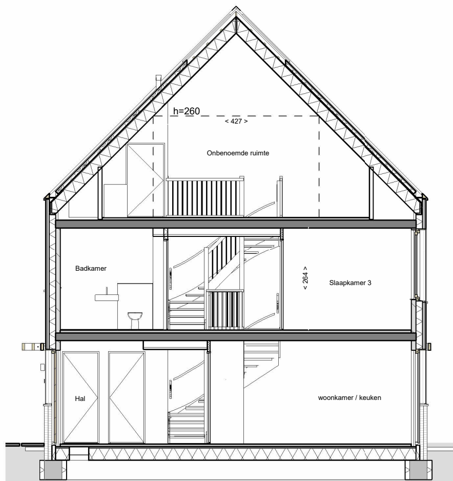
doorsnede
