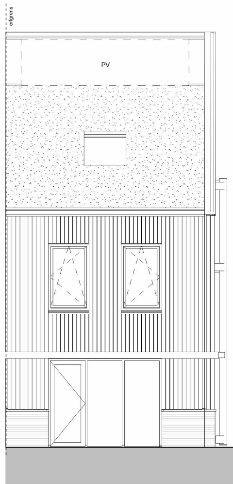
achtergevel
