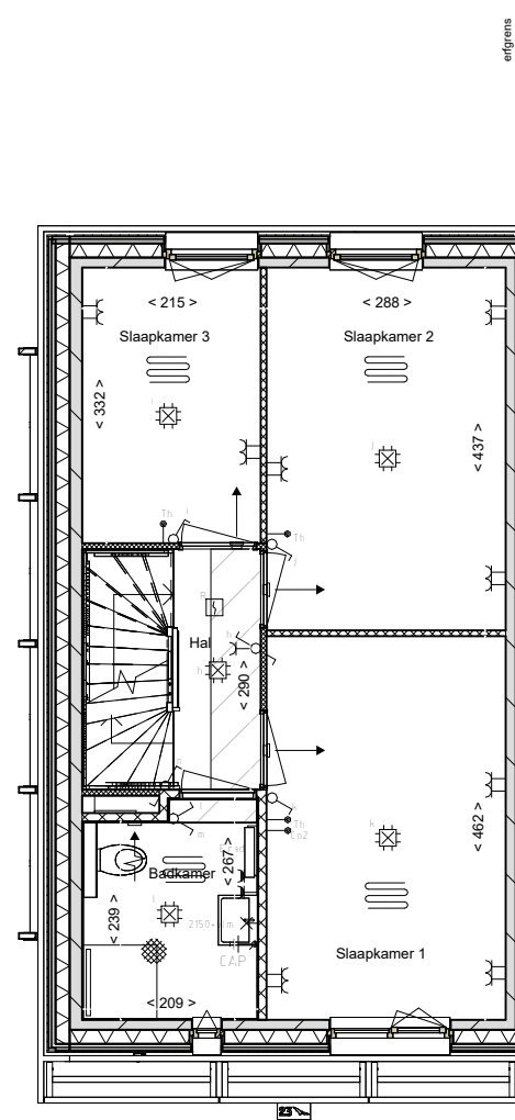
01 eerste verdieping
